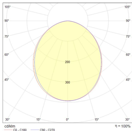
Ultralim 36W
