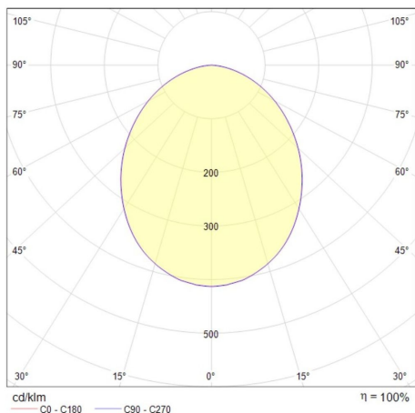
Ultralim 48W
