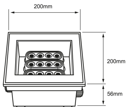
Uplight 19.5W Cuadrado
