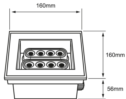
Uplight 13.5W Cuadrado
