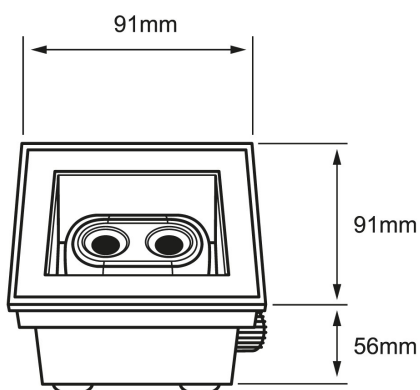
Uplight 5.5W Cuadrado
