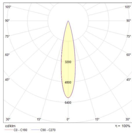
Uplight 13.5W Cuadrado
