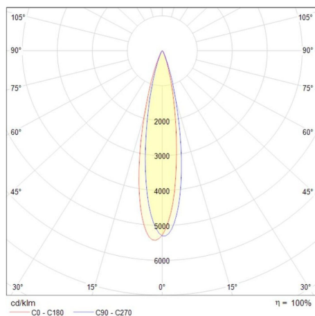
Uplight 5.5W Cuadrado
