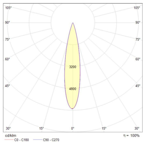
Uplight 19.5W Cuadrado
