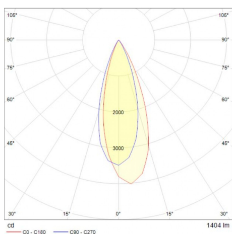
Trazzo Grazer Dirigible 20W
