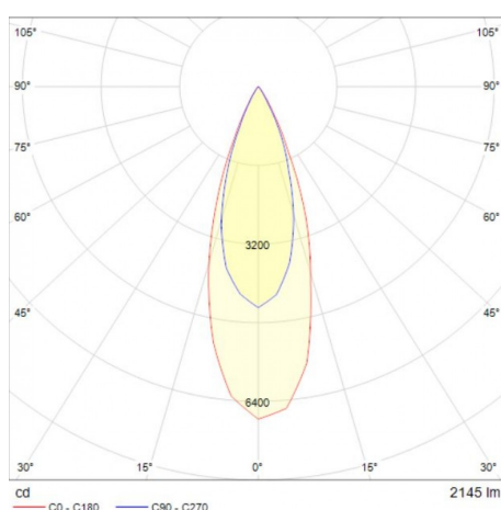
Trazzo Grazer Dirigible 30W
