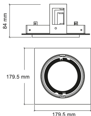
Modulare 17W AR111
