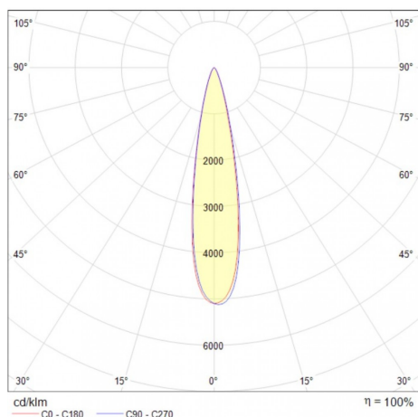
Modulare 17W AR111 24°
